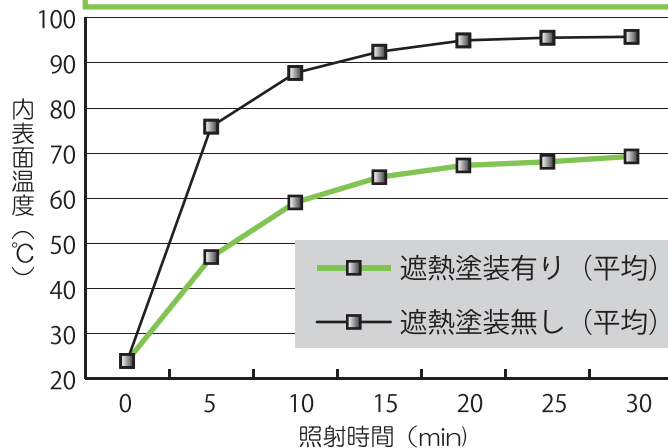
ST#157 型の遮熱塗装有無による遮熱効果比較
