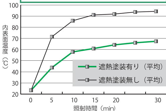
ST#101 型の遮熱塗装有無による遮熱効果比較
